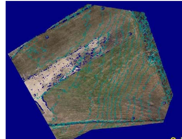
Relieve y microrrelieve del terreno
